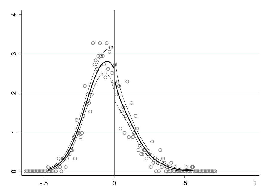
Gráfico 4: Prueba McCrary de discontinuidad de la variable de tratamiento
